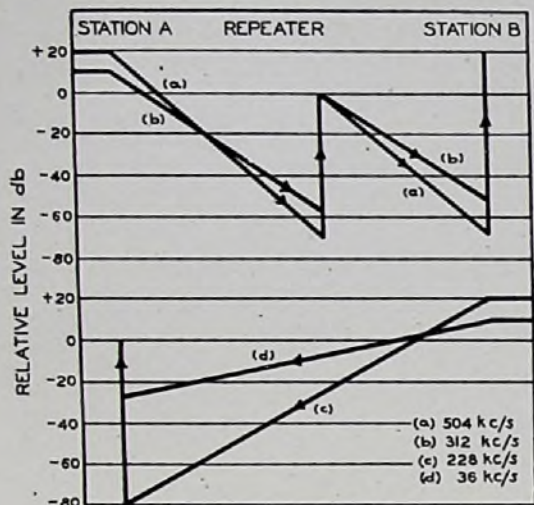
FIG. 3.—LEVEL DIAGRAM.
