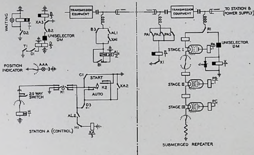
FIG. 7.—SWITCHING CIRCUIT.
