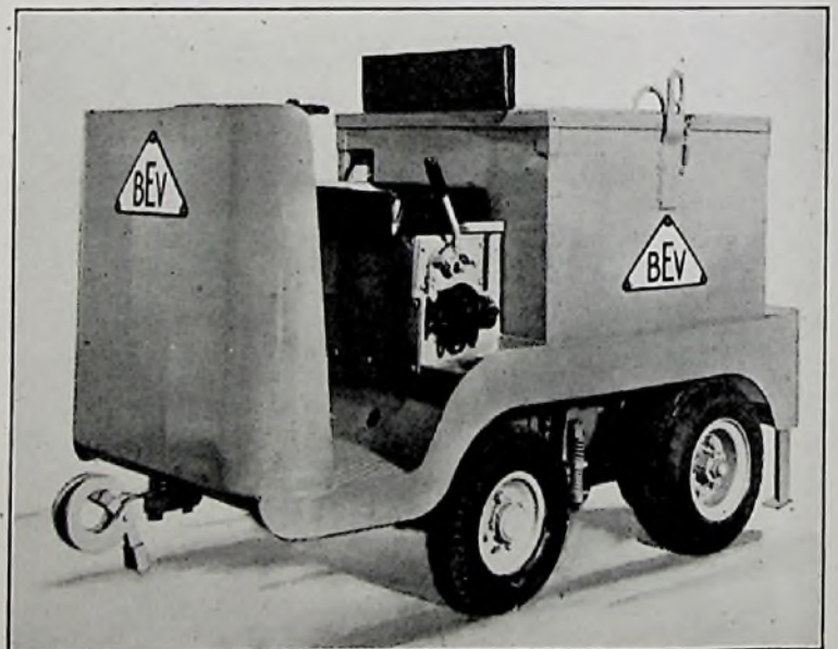
FIG. 4.—"B.E.V." TRACTOR.
