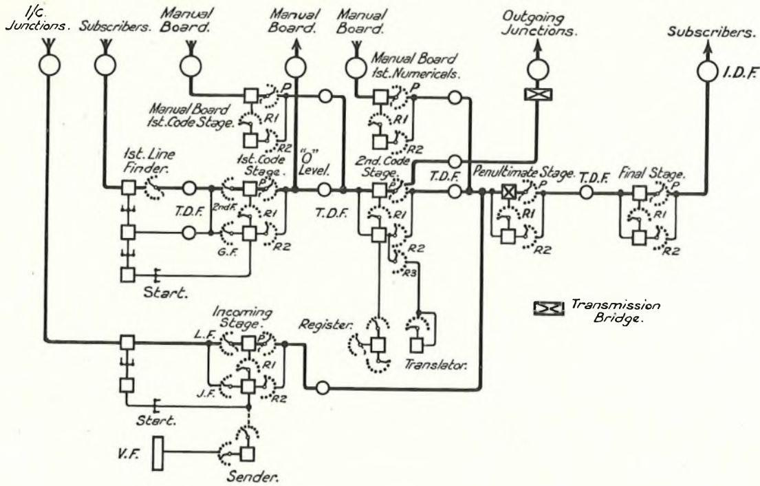
FIG. 2.—KEY DIAGRAM.
