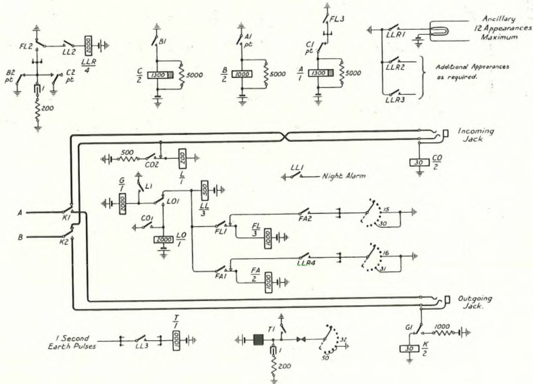
FIG. 7.—BOTHWAY PHONOGRAM CIRCUIT.
