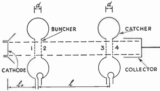
Fig. 1—Diagram of klystron
