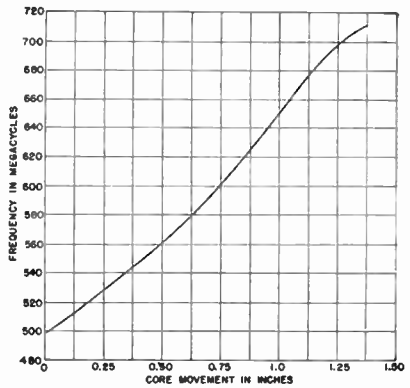
Fig. 11—Tuning curve.
