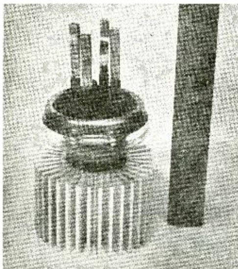
Fig. 1—The RCA-827R.
