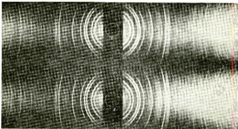
(a) \alpha\text{-ZnO}\cdot\text{SiO}_2 . 1200 °C — 2 Hours (b) \alpha\text{-ZnO}\cdot\text{SiO}_2 . 1200 °C — 1 Hour
