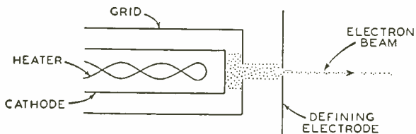
Fig. 6—Electron gun.
