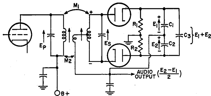
Fig. 33—Ratio-detector circuit.
