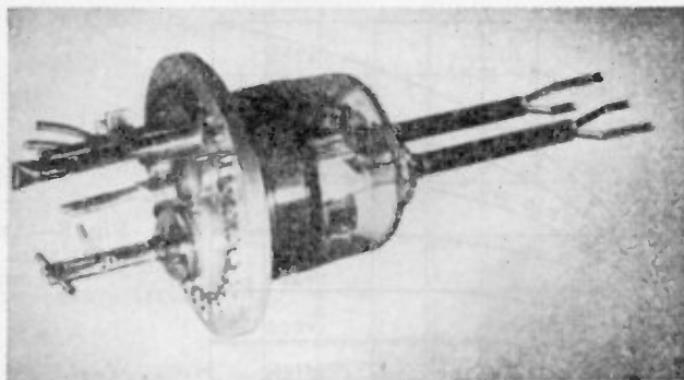
Fig. 7—The duplex tetrode.
