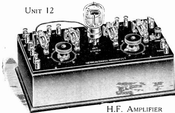
H.F. AMPLIFIER
