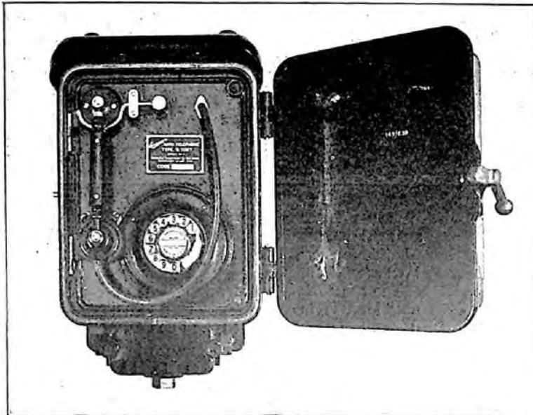
FIG. 1.—TELEPHONE No. 149—ACCESS DOOR OPEN.
