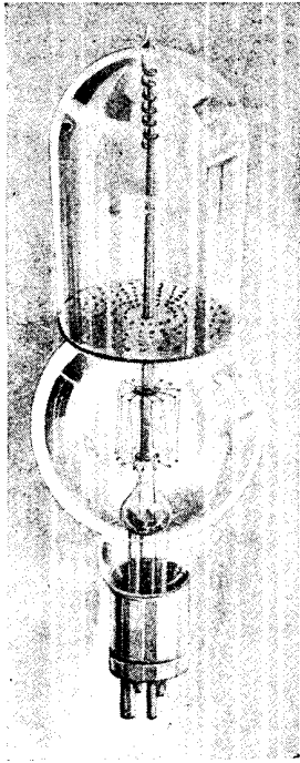
LIEBEN-REISZ VALVE
