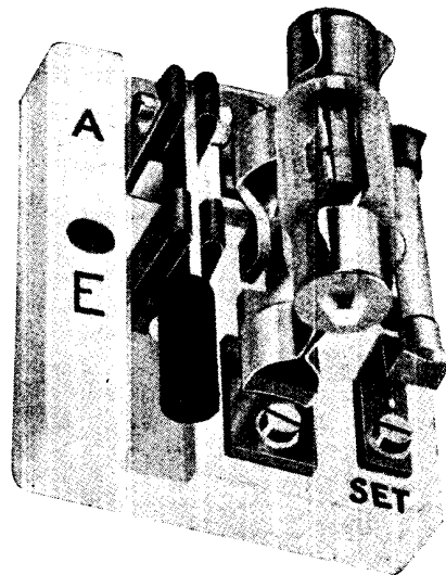
SIEMENS LIGHTNING ARRESTER
