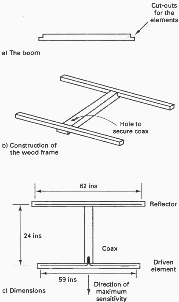
Fig. 4.4 Simple VHF FM Yagi.
