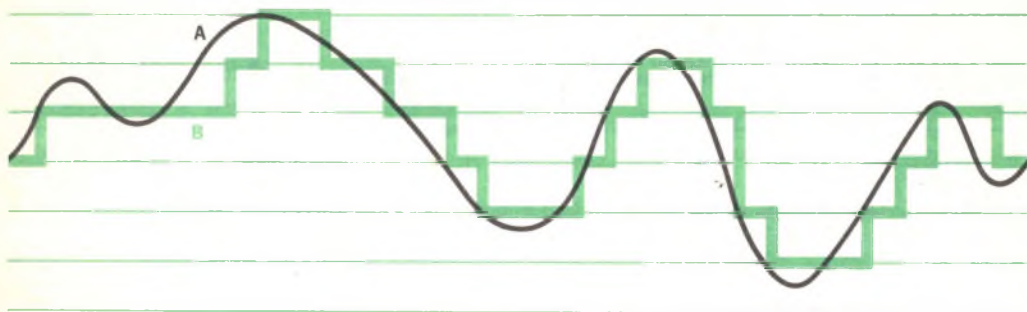
La forma d'onda a scalini B si ottiene dalla forma d'onda continua A quantizzandola su sette livelli equidistanti. L'area ombreggiata rappresenta l'errore di quantizzazione e può essere ridotta introducendo un maggior numero di livelli, meno distanti l'uno dall'altro.
