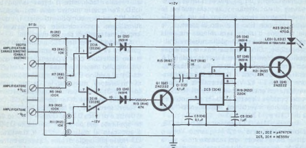
Fig. 2 - Schema del circuito indicatore di tosaturo per un canale.
