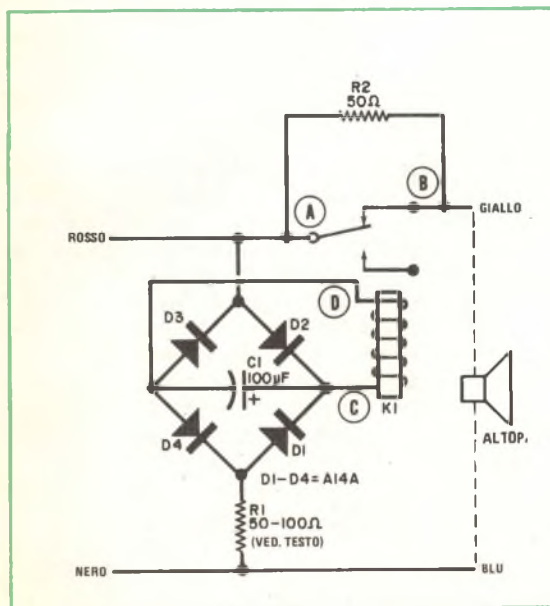
Fig. 1 - Il circuito autoalimentato riduce automaticamente il livello degli altoparlanti quando sopraggiungono picchi di potenza.
