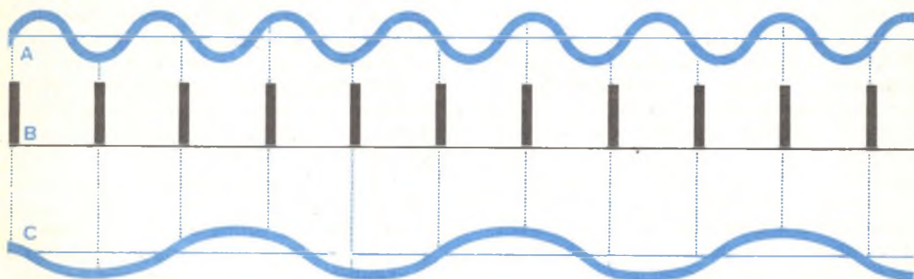
Distorsione di ribaltamento (aliasing): la sinusoide A (in alto) ha una frequenza maggiore della sequenza di impulsi B, usata per il campionamento. La sinusoide C, con frequenza più bassa di A, dà la stessa serie di campioni ed è quella che compare all'uscita quando il segnale campionato viene ricostruito.
