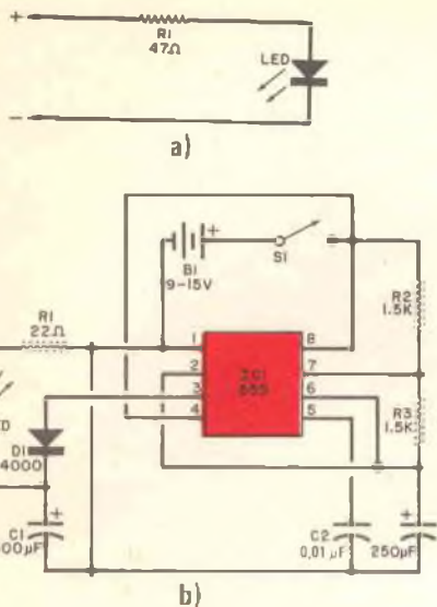
Fig. 2 - Semplice provabatterie con LED policromo (a), e circuito lampeggiatore con LED policromo (b).
