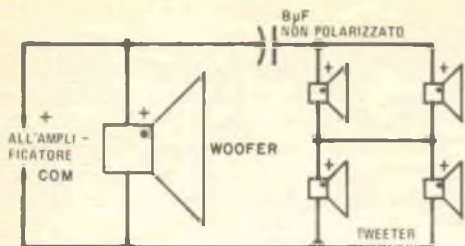
Fig. 4 - Schema di collegamento degli altoparlanti: si noti l'uso del condensatore.
