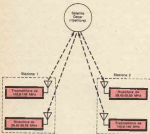
Fig. 3 - Sistema base per comunicazioni "auto patch" per la banda per amatori del 2 m.
