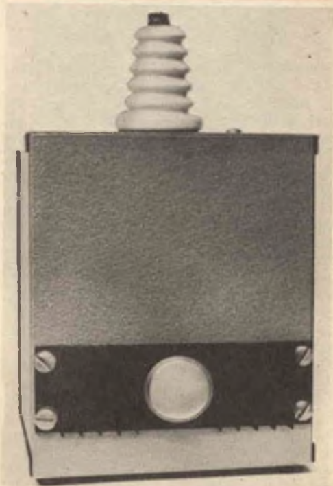
Fig. 5 - Il transistor è elettricamente isolato dal radiatore di calore e questo è fissato alla parte posteriore della scatola. L'involucro (collettore) di Q1 non deve entrare in contatto con parti metalliche.
