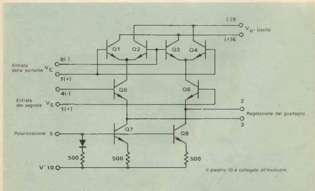
Fig. 2 - Schema del modulatore/demodulatore Motorola MC1596/1496
