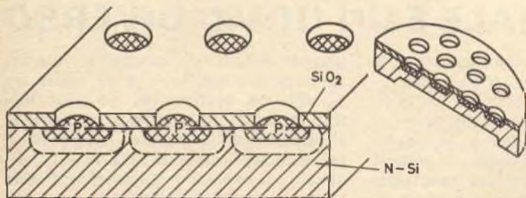
Struttura di un target di silicio vista in prospettiva.
