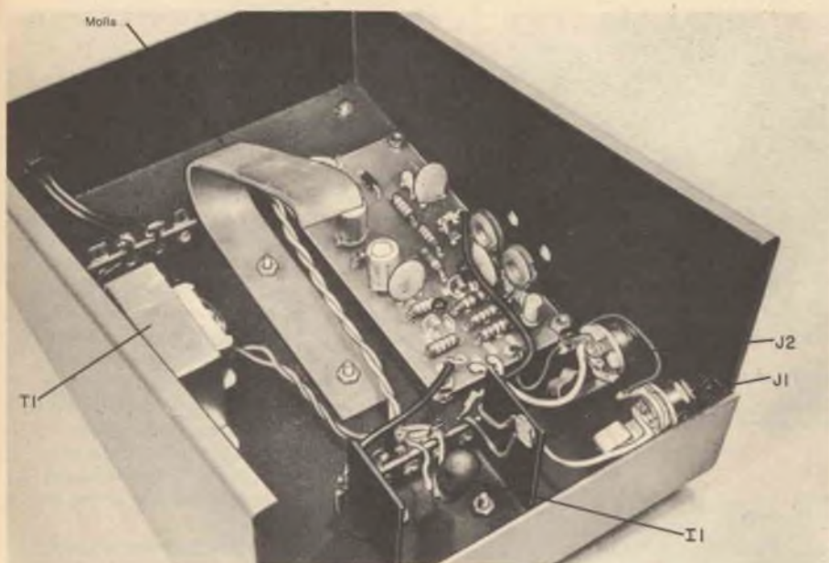
Veduta interna del dispositivo da cui è visibile la posizione di tutte le parti. Si notino i due fori per i potenziometri di regolazione. I bordi ripiegati del telaio limitano la curva verso l'alto del pedale.
