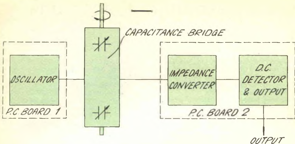
Schema dell'elemento trasduttore realizzato dalla Jackson Brothers (London) Ltd.
