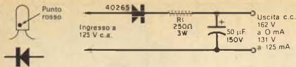
Fig. 4 - Questo generatore di segnali a mezz'onda impiega un raddrizzatore al silicio 40265 da 400 V - 125 mA, equivalente al tubo 35W4.
