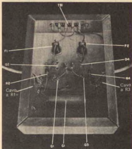
Fig. 3 - Ecco la parte inferiore del telaio: risulta chiaramente visibile la disposizione dei componenti e dei collegamenti. Il condensatore C1 è collegato all'uscita del gruppo trasformatore raddrizzatore in modo da fornire una corrente continua filtrata agli amplificatori. Fate uso di gommini passafilo per i fori di uscita dei cavi.
