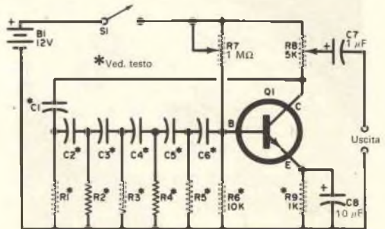
Fig. 2 : Oscillatore BF a rotazione di fase adottato per essere usato come oscillafono.
