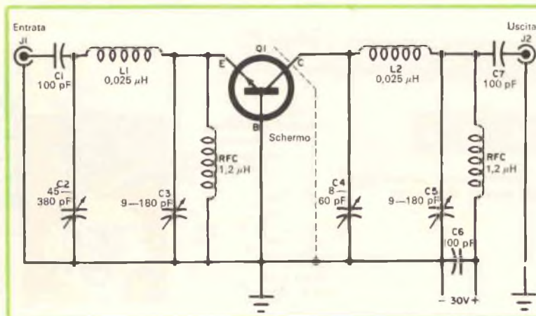
Fig. 1 - Ecco un amplificatore di potenza in classe C a 160 MHz, progettato dalla Texas Instruments. La potenza d'uscita è di 750 mW e la lunghezza di banda di 15 \text{ MHz} \pm 3 \text{ dB} .
