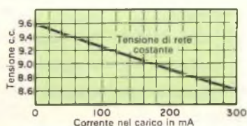
Tensione d'uscita in funzione della corrente nel carico.
