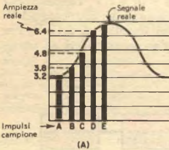
Fig. 4 - Nel sistema a modulazione ad impulsi codificati, l'ampiezza del segnale reale (A) è campionata a intervalli regolari; i segnali campione sono arrotondati in un numero intero rappresentando l'ampiezza dell'impulso, cioè in un segnale quantizzato (B), e quindi convertiti in numeri binari. Lo schema del codice binario (C) dà il valore decimale corrispondente ai numeri binari.
