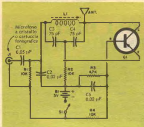
Fig. 3 - Costruito per essere impiegato con cartucce a cristallo di uscita moderata o elevata, questo oscillatore è regolato in modo da irradiare un segnale in un angolo morto della banda delle onde medie mediante la bobina L1 a nucleo di ferrite regolabile.
