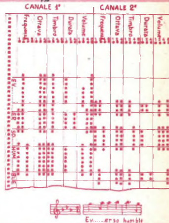
Fig. 6 - Carta di registrazione a perforazione del sintetizzatore a due canali indipendenti. La frase EVER SO HUMBLE, registrata con questo sistema, è stata ripetuta in basso con le notazioni convenzionali. L'allineamento dei fori superiori punzonati a solo titolo di riferimento dà l'indicazione del numero di combinazioni, secondo il sistema binario, assegnato ad ognuno delle caratteristiche del suono per la segnalazione di tutti i circuiti interessati.
