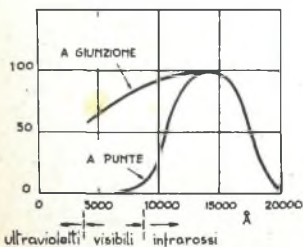
Fig. 16 - Caratteristica di sensibilità di fototransistori.
