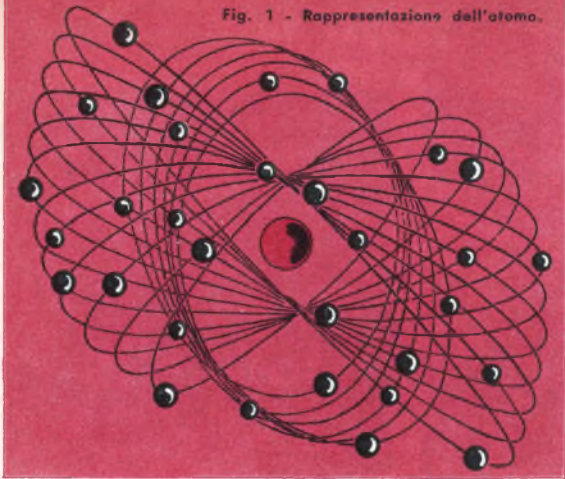
Fig. 1 - Rappresentazione dell'atomo.
