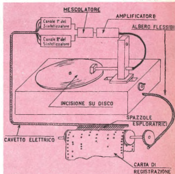
Fig. 7 - La serie delle spazzole esploratrici, passando sui fori delle carte di registrazione, predispongono nel sintetizzatore i vari circuiti per la generazione di due distinti ed indipendenti segnali di uscita: Canale 1° e Canale 2° che nel mescolatore danno luogo ad un segnale risultante adeguatamente amplificato prima di comandare il registratore.
