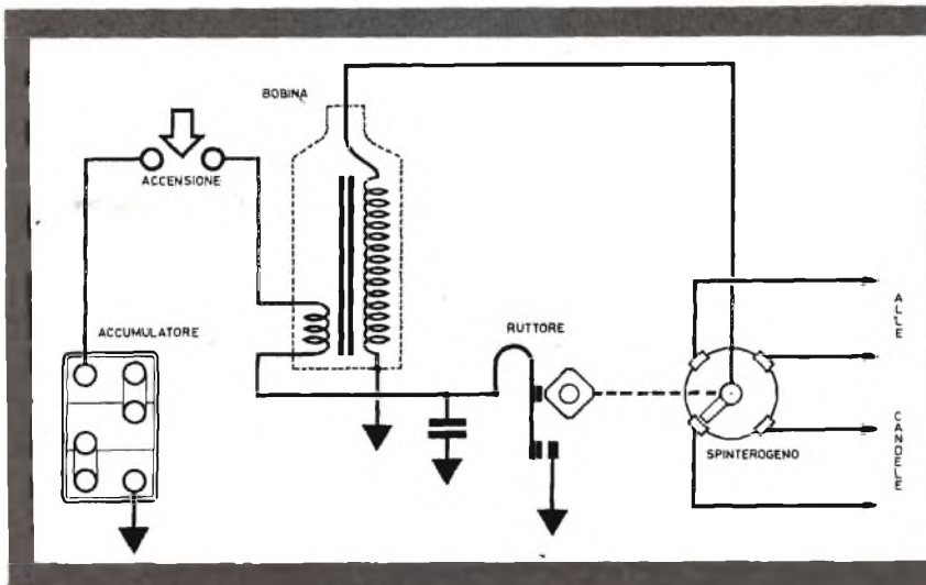
Fig. 1 Nello schema in figura è rappresentata quella parte dell'impianto elettrico di un'automobile che è principalmente la fonte dei disturbi radioelettrici, quella su cui occorre intervenire nel modo descritto in queste pagine.
