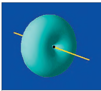
4 – L'antenne demi-onde dans l'espace.
