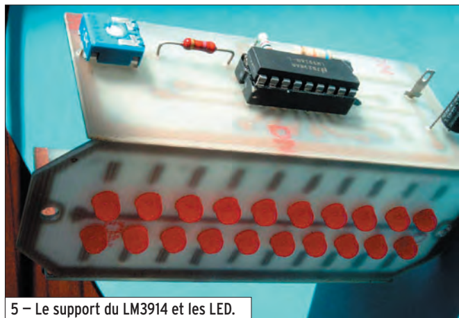
5 – Le support du LM3914 et les LED.
