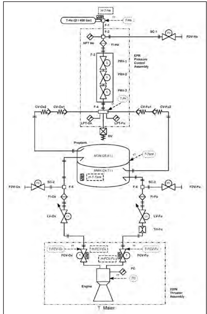
12 - Vue synoptique du système de propulsion de P3E.
