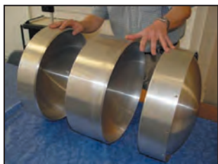
7 - Montage du réservoir d'hélium.
