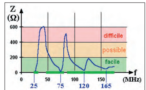
Figure 8: Possibilité d'accord de l'antenne sur une bande de fréquence.
