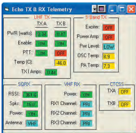
Figure 8 : Emetteurs / Récepteurs en fonctionnement.
