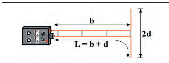
Figure 3 : Antenne center-fed de laboratoire.
