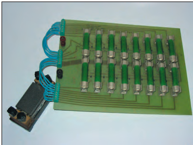
Photo 7 : La charge utilisée pour les essais. Elle est réalisée avec 16 résistances de 12 ohms en parallèle sur une plaque de circuit imprimé. Chaque résistance peut dissiper 32 watts en régime permanent. Cette charge permet de tester les alimentations jusqu'à 19 volts et 25 ampères. Le shunt à côté de la charge est un 20 A / 50 A - 0,1 V ; il est utilisé pour mesurer le courant de sortie de l'alimentation.
