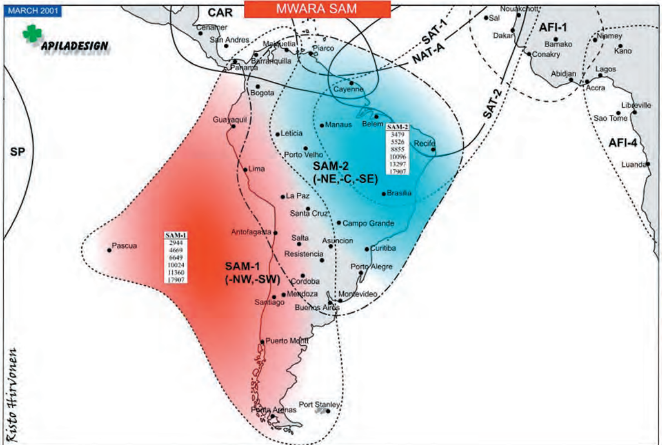
Résumé des fréquences MWARA (en kHz) apparaissant sur les cartes publiées dans MEGHERTZ magazine
