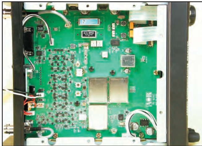
Une vue du circuit imprimé principal supportant les filtres FI.
