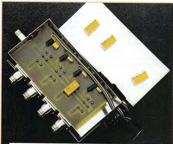
La boîte et ses relais. Notez les connecteurs de qualité (ici, des NJ) et surtout, le tore de ferrite destiné à bloquer la HF vagabonde.
