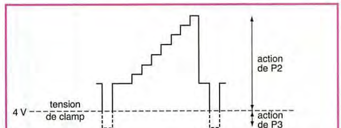
Figure 6 : P3 fait descendre les tops synchro au-dessous du seuil de clamping ; P2 agit sur l'amplitude du signal composite d'origine
