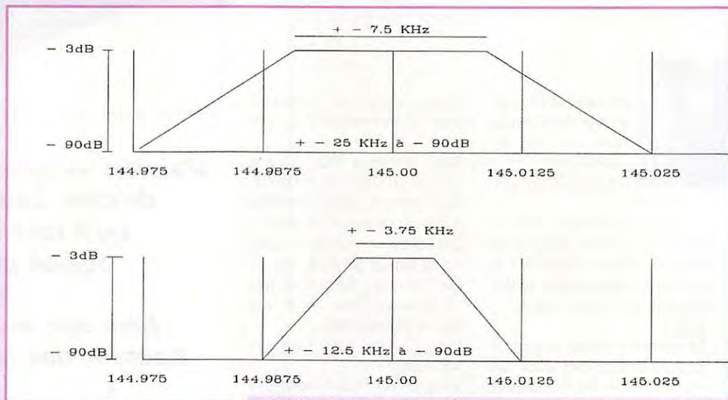
Schématisation de la bande passante d'un filtre à quartz 8 pôles pour une grille de fréquences à 25 kHz et 12,5 kHz.
