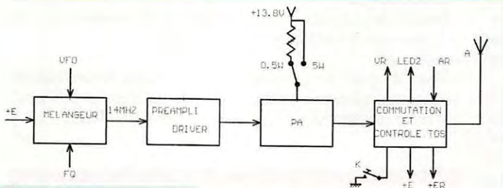
Figure 14 : Synoptique Emetteur.
