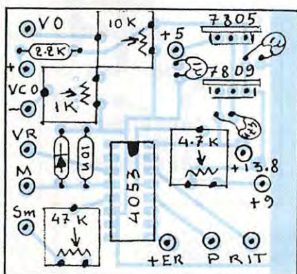
Figure 20 : Implantation Auxiliaires.
