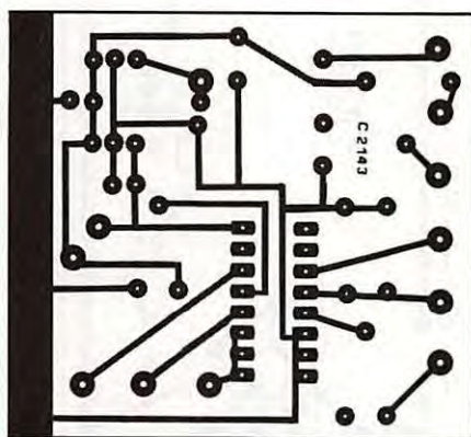
Figure 19 : C.I. Auxiliaires.
