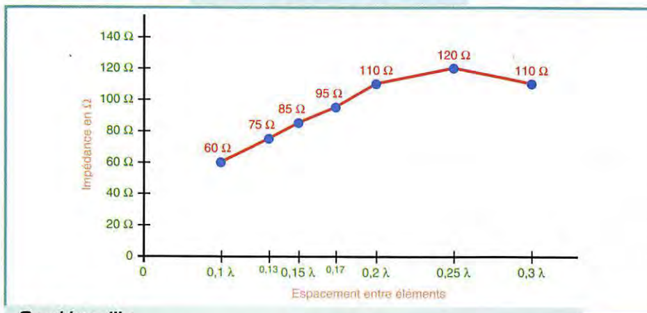
Graphique III : Impédance d'un cadre selon l'espacement d'un élément parasite.
