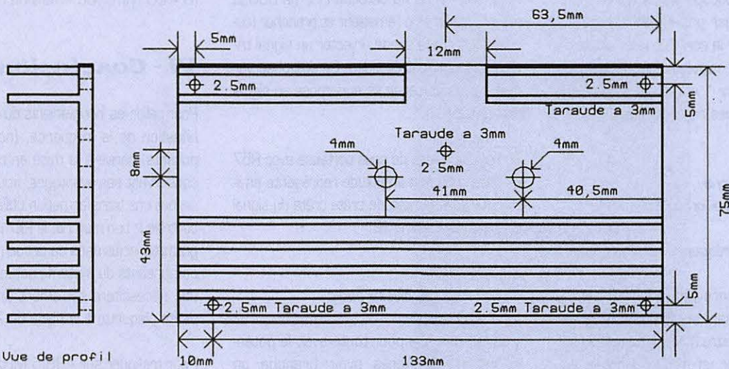
Figures 10-11. Plan de perçage radiateur. En haut : version 1. En bas version 2.
