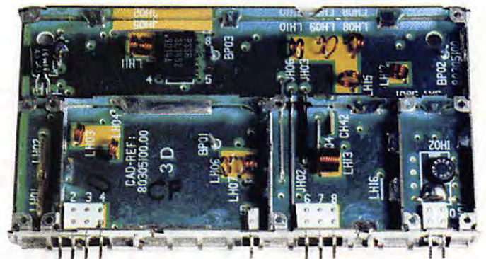
Le module tuner est livré monté et réglé.
