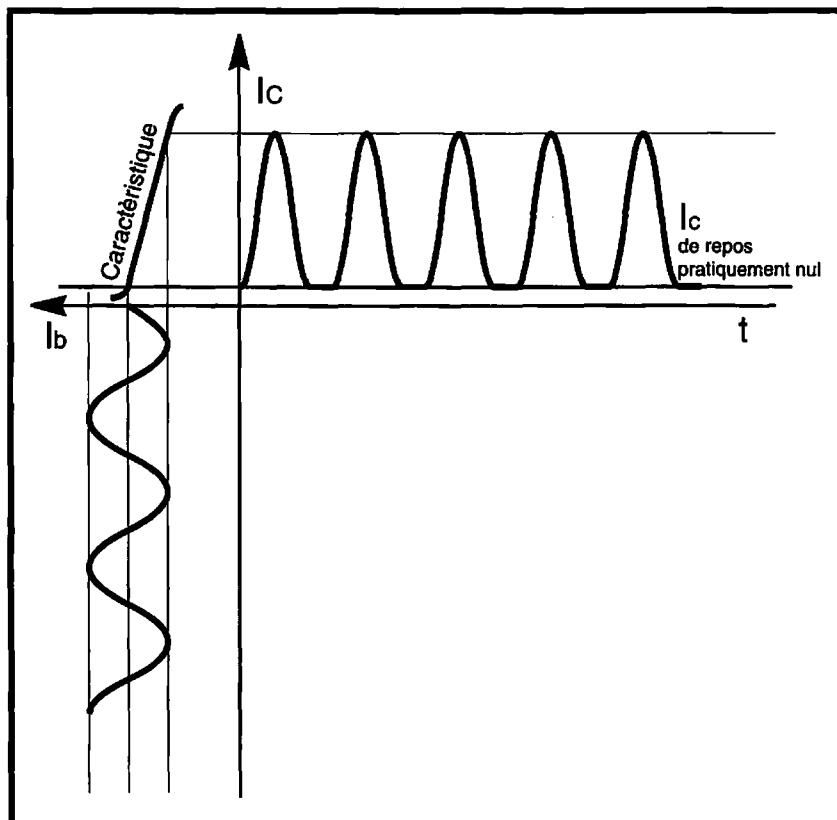
Fig. 4 - L'amplification en classe B.
