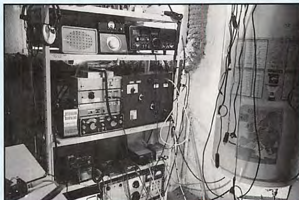
F10K : la station.
