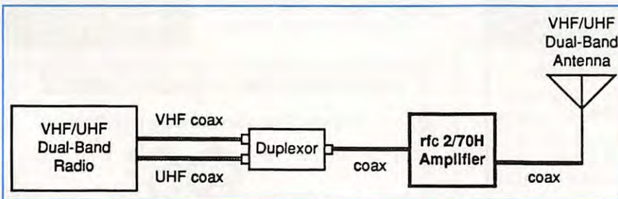
Duplexeur indispensable devant cet ampli bibande.
