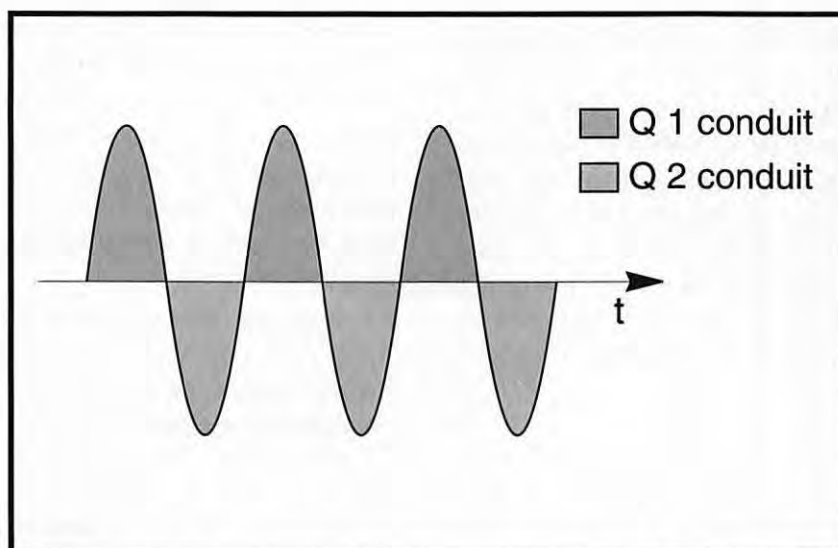
La conduction de deux transistors montés en push-pull et polarisés en classe AB1 ou AB2.
