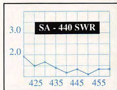
Courbe de TOS du constructeur ; elle peut varier suivant l'installation. L'antenne couvre de 425 à 480 MHz.
