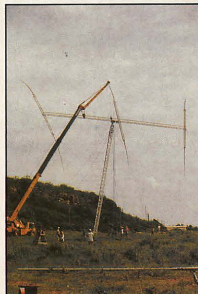
Montage de l'antenne 80 m avec une grue.
