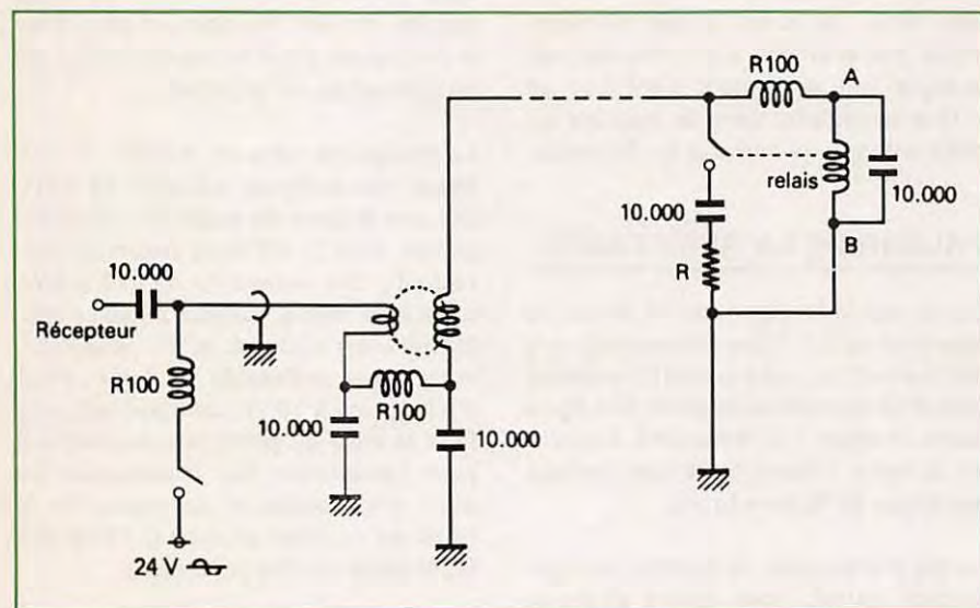
Figure 6a : Télé-commutation de la résistance placée en bout de fil. La partie relais entre A et B peut être modifiée comme indiqué sur la figure 6b en cas d'utilisation d'un relais exigeant une tension continue.
