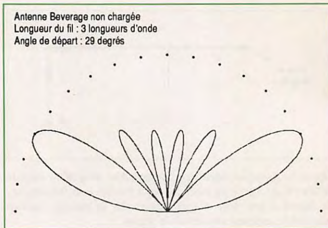
Figure 5 : Diagramme de rayonnement dans le plan vertical d'une antenne Beverage à extrémité libre ; ( l = 3 \lambda ).
