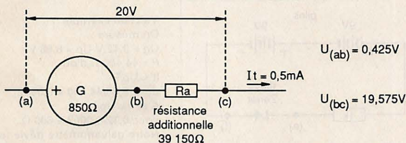
Figure 3 : Utilisation d'un galvanomètre en voltmètre
