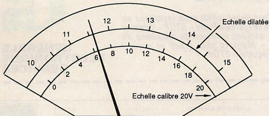
Figure 4 : Graduations de l'échelle dilatée
