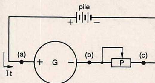
Figure 1 : Définition des caractéristiques d'un galvanomètre
