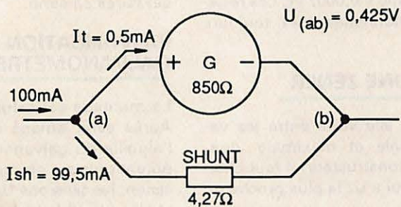
Figure 2 : Utilisation d'un galvanomètre en ampèremètre
