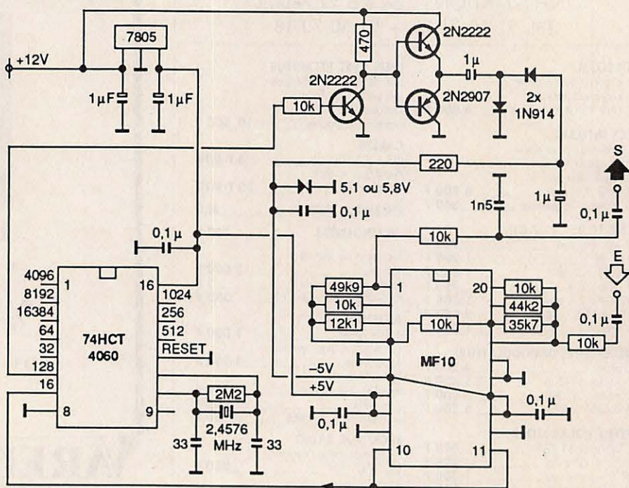
E = Entrée Audio S = Vers PK1, broche 2 du XR2211 (sans rien d'autre)
