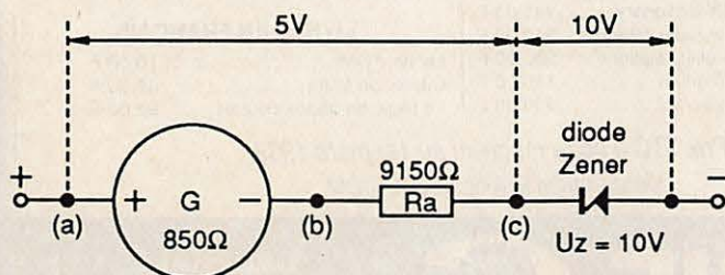
Figure 5 : Réalisation électronique de la dilatation d'échelle
