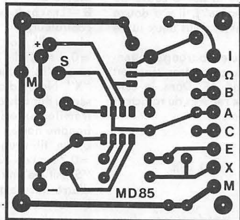
Figure 1 Le circuit électronique s'appuie sur un ampli opérationnel BI-FET monté en amplificateur direct de tension.
