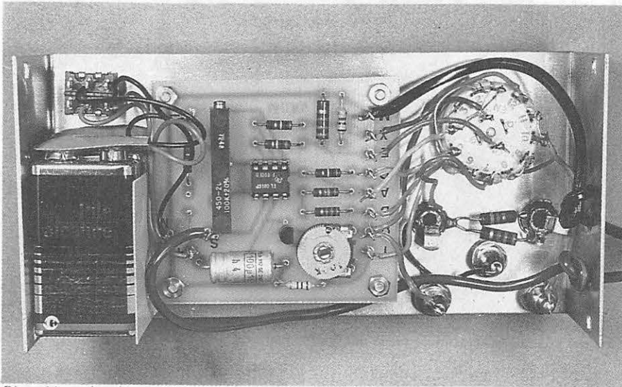
Dispositions des divers éléments dans le coffret TEKO 41B.
