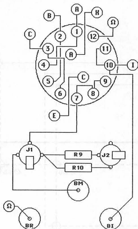
Figure 4 Câblage du rotacteur et des socles.
