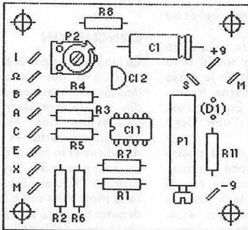
Figure 2 Le circuit imprimé est représenté grandeur nature.
