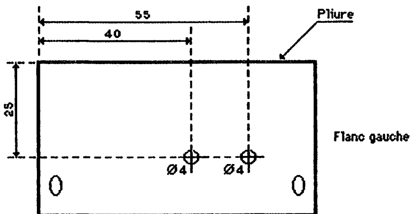
Figure 3 Plan de perçage en vues externes du couvercle du coffret TEKO 4/B.
