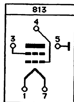
brochage du tube
