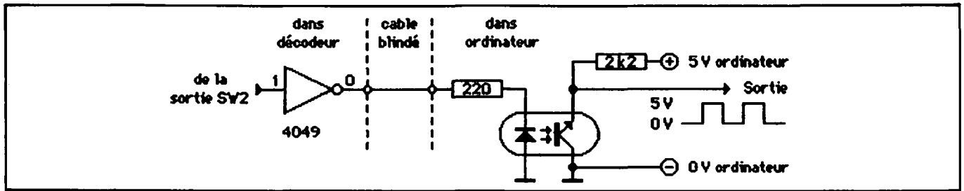
Commande par optocoupleur.
