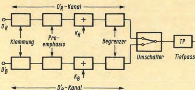
Bild 2. Blockschaltbild für die niederfrequente Aufbereitung der FD-Signale
