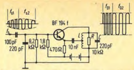
Bild 8. Prinzip eines mitgezogenen Oszillators. Die Oszillatorknotenfrequenzen f_{01} und f_{02} werden durch die Steuerfrequenzen f_{s1} und f_{s2} synchronisiert
