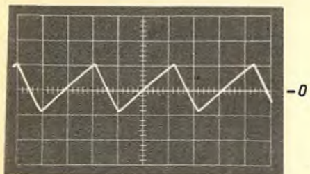
Bild 5. Spannung am Emittter des Transistors T 1. Maßstab: vertikal 1 V/T, horizontal 20 \mu s/T
