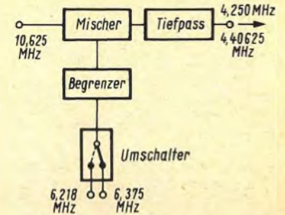
Bild 9. Blockschaltbild des Umsetzers
