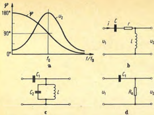
◀ Bild 3. a = Amplituden- und Phasengang von Schwingkreisen in Vierpolanordnung. Bei der Resonanzfrequenz f_0 beträgt der Phasenwinkel der Ausgangsspannung 90^\circ ; b = Serienschwingkreis als Vierpol; c = Parallelschwingkreis mit kleinem Vorschaltkondensator C_1 als Vierpol; d = Ersatzschaltung zu Bild 3c
