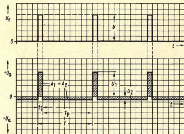
Bild 5.2. Kapazitive Kopplung einer Rechteckimpulsfolge mit dem Tastverhältnis V = 10
