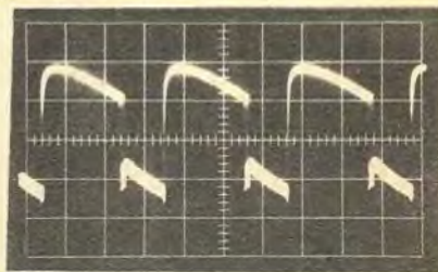
Bild 17. Zeilenfrequenter Anteil der Ausgangsspannung des Netzteiltes bei 80 W Belastung. Maßstab: vertikal 1 V/T, horizontal 20 \mu s/T
