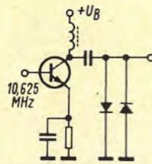
Bild 8. Schaltung eines einfachen Begrenzers
