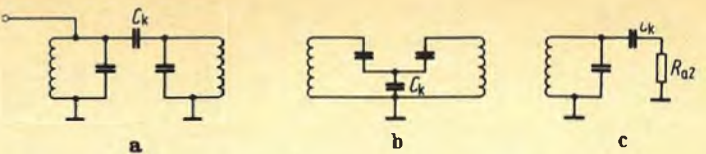
▲ Bild 5. a und b = kapazitiv gekoppelte Bandfilter; c = Ersatzschaltung
