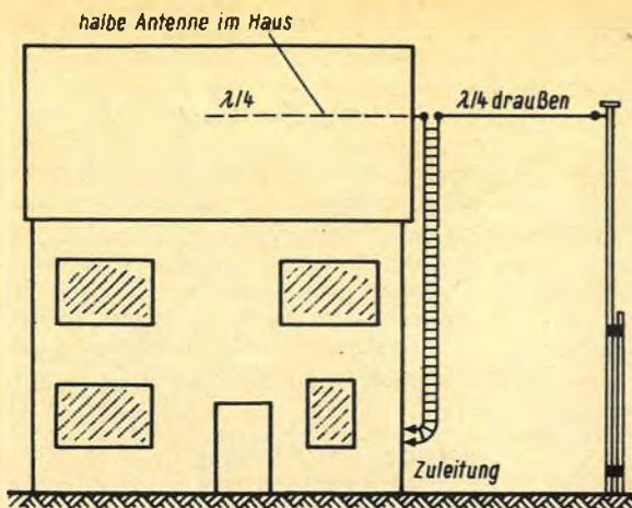
◀ Bild 8. Dipolantenne, teilweise im Dachboden verspannt
