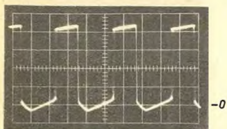
Bild 6. Spannung am Kollektor des Transistors T 1. Maßstab: vertikal 2 V/T, horizontal 20 \mu s/T
