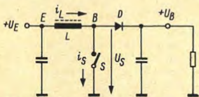
Bild 1. Prinzipschaltung des Netzteiles
