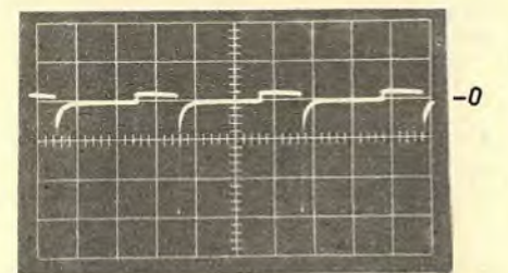
Bild 9. Gate-Strom des Thyristors GTO. Maßstab: vert. 1 A/T, horiz. 20 \mu s/T [neg. Spitzenwert = 3 A]
