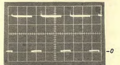
Bild 10. Spannung an der Anode des Thyristors GTO. Maßstab: vert. 100 V/T, horiz. 20 \mu s/T
