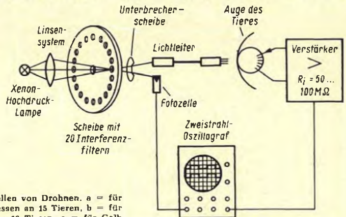
Bild 2. ► Meßeinrichtung zum Bestimmen der Farbeempfindlichkeit von Sehzellen
