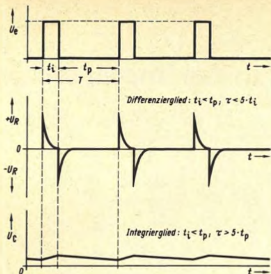
Bild 4.11. Rechteckimpulsfolge mit t_i \neq t_p ; Dimensionierung der Zeitkonstante beim Differenzglied und beim Integrierglied
