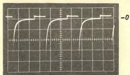
Bild 8. Spannung am Gate des Thyristors GTO. Maßstab: vertikal 5 V/T, horizontal 20 \mu s/T
