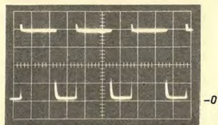
Bild 7. Basisspannung von Transistor T 3. Maßstab: vertikal 1 V/T, horizontal 20 \mu s/T
