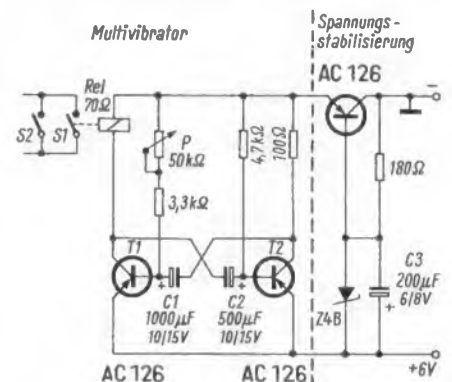
Mit dem kleinen Zusatzgerät für die Scheibenwischanlage lassen sich verschieden lange Pausen zwischen den Wischvorgängen einstellen
