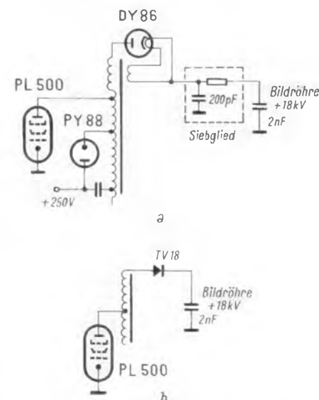
Bild 8. Zeilen-Endstufe eines Schwarzweiß-Fernsehempfängers mit Hochspannungsgleichrichterröhre DY 86 (a) und mit Selen-Stabgleichrichter des Typs TV 18 (b)
