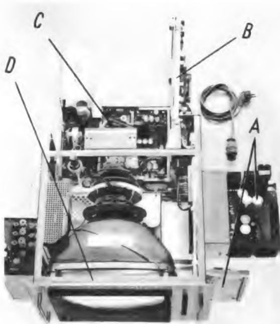
Bild 1. Die herausklappbaren Baugruppen des Farbfernseh-Monitors MF-01 (Erklärungen siehe Text)
