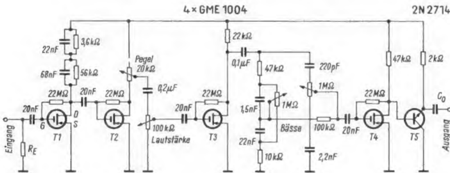
Bild 3. Schallplatten-Vorverstärker mit Entzerrgliedern
