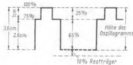
Bild 2. Kontrolle des Signal/Impuls-Verhältnisses des Bildsignals auf dem Oszillografenschirm bei einer eingestellten Impulshöhe von 3,6 cm
