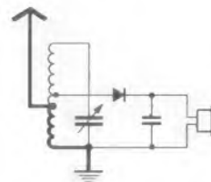
Bild 5.4. Induktive Ankopplung der Antenne mittels Spartransformator
