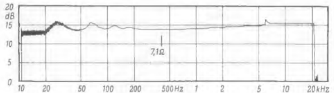
Bild 3. Impedanzverlauf der Schwingspule des Lautsprechers P 21/25/11 in der Exponentialbox
