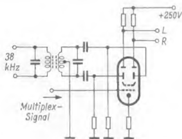
Bild 9. Decodierung mit strahlabgelenkter Pentode[5]
