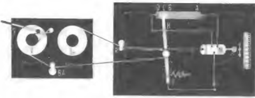
Bild 3. Das Prinzip des Synchronisier-systems. Es bedeuten im Projektor: A - B = Widerstandsbahn, C = Halbstellung, D = Rücklauf, F = Spannfeder, H = Fühlhebel, M = Motor, R = Transportrolle; im Tonbandgerät: BA = Andruckrolle, V = Vorratsspule, Sp = Aufwickelspule
