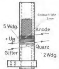
Bild 7. Wickelanordnung der Oszillatorspule
