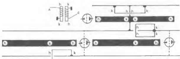
Bild 3. Koppelprinzip „heiß an kalt“; h = heiße Punkte, k = kalte Punkte
