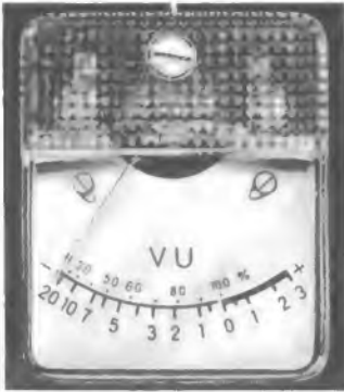
Bild 1. Ansicht eines Volumen-Meters aus dem Gerät Revox G 36
