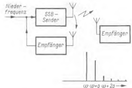
Bild 6. Eine einfache Modulationsmethode für CSSB
