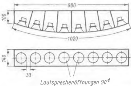
Bild 6. Baumaße für das MH-Gehäuse. Die Außenwände bestehen aus 1,8 mm starkem Sperrholz, die Trennwände und die Rückwand aus Weichfaserplatten
