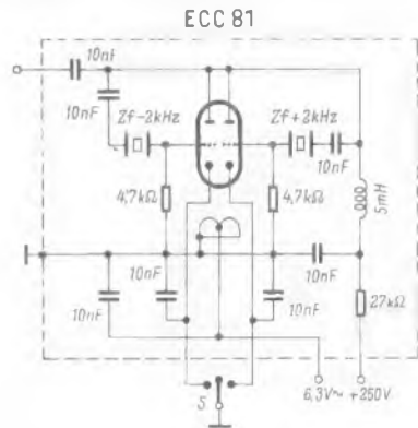
Schaltung eines Kristallüberlagerers für das obere und das untere Seitenband durch getrennte Kristalloszillatoren
