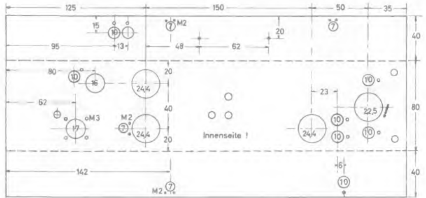
Bild 17. Chassisabmessungen
