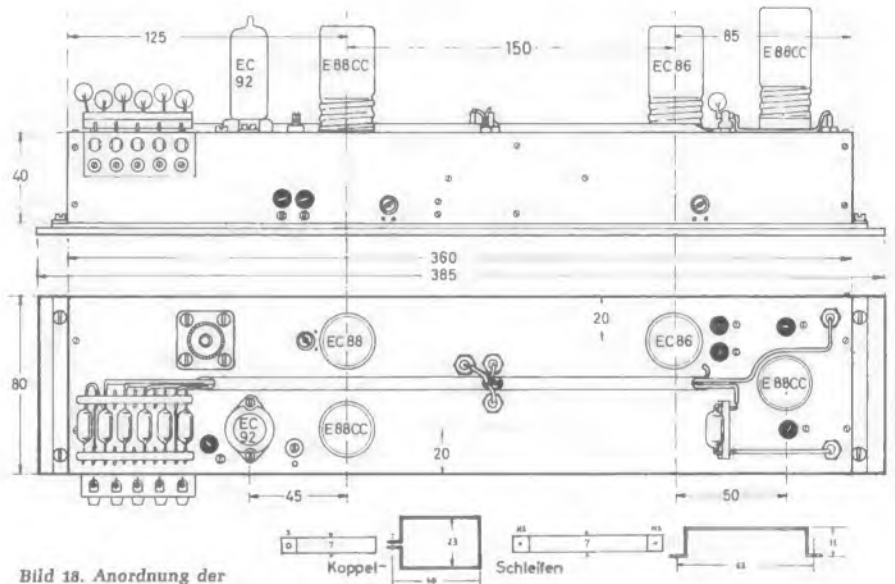
Bild 18. Anordnung der Bauteile auf dem Chassis
