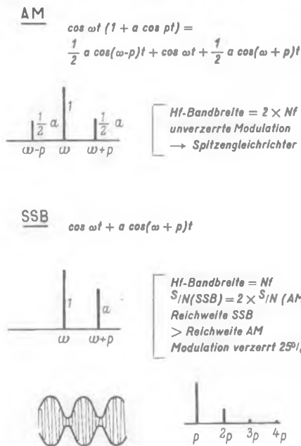
Bild 5. Vergleich von Amplitudenmodulation und Single Sideband Modulation (AM und SSB)
