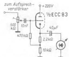
Bild 3. Gesamtschaltung eines VU-Meters
