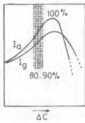
Bild 8. Arbeits- punkteinstellung des Oberton- Oszillators
