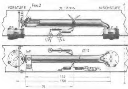
Bild 11. Konstruktion des \pi -Kreises
