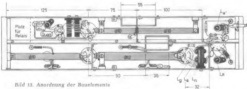
Bild 13. Anordnung der Bauelemente
