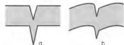
Bild 5. Richtige Form der Bild-Austastimpulse am Wehneltzylinder (a); bei einem fehlerhaften Impuls (b) erscheint der Bildschirm im oberen Drittel dunkler
