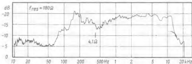
Bild 8. Schalldruck-Frequenzverlauf eines Einzelsystems P 10/Cl-13/65-10000e Cu mit Dämpfungstegen
