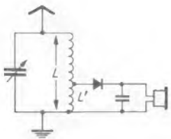
Bild 5.1. Detektor-Empfänger mit Anpassung des Verbrauchers an den Schwingkreis
