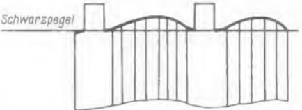
Bild 4. Bei Brummeinstreuungen erscheint der Schwarzpegel verzogen
