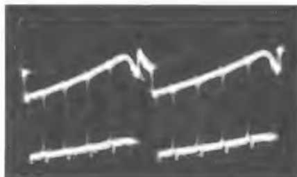
Bild 11. Oszillogramm des Fehlers nach Bild 10 an der Katode der Bildröhre mit verzogenem Schwarzpegel und einer Dachschräge des Zeilen- impulses
