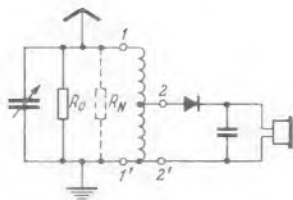
Bild 5.2. Empfänger nach Bild 5.1 mit eingezeichnetem Resonanzwiderstand R_0 und übersetztem Verbraucherswiderstand R_N
