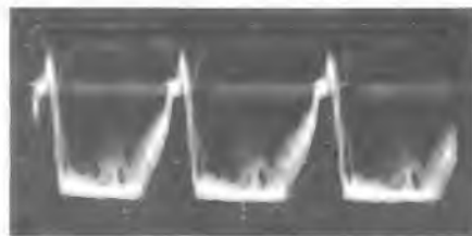
Bild 7a. Bei einem Fehler nach Bild 7 ist ein völlig deformiertes Signal an der Katode der Bildröhre zu messen
