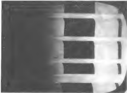
Bild 10. Fehlerhaftes Schirmbild auf Grund mangelhafter Kapazität des Siebkondensators der getasteten Regelung. Die Synchronisation der Kipp- teile ist hierbei labil
