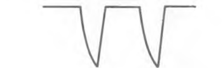
Bild 6. Form der Zeilen-Austastimpulse an der Bildröhre
