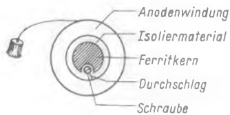
Ein Durchschlag von der Anodenwicklung zur Schraube, die den Kern des Zeilentransformators zusammenhält, ergab einen Masseschluß
