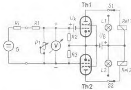
Bild 1. Das Prinzip eines Grenzwertschalters
