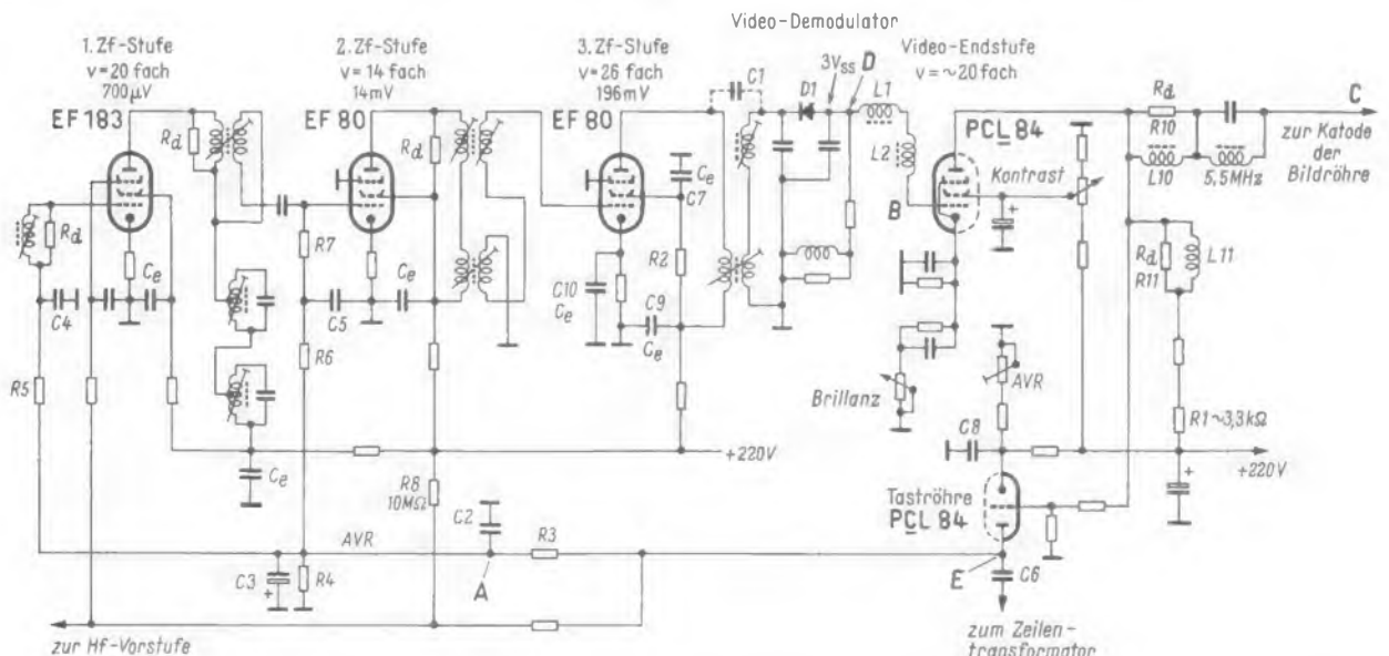
Bild 1. Schaltung eines Zf-Verstärkers mit Video-Demodulator und Video-Endstufe. V bezeichnet die Verstärkungsfaktoren der einzelnen Stufen. Um am Video-Demodulator eine Spannung von 3 V_{88} zu erhalten, müssen den Zf-Stufen die dort vermerkten Spannungen vom Signalgenerator zugeführt werden
