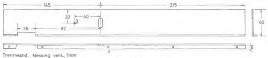
Bild 16. Maße der Trennwand
