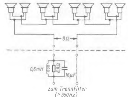
Bild 4. Schaltung der MH-Lautsprecher und des Parallelschwingkreises zur Dämpfung von Schalldrucküberhöhungen im Bereich um 2 000 Hz
