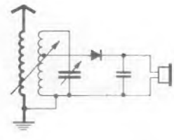
Bild 5.5. Antennenanpassung mittels getrennter, induktiv mit der Schwingkreis-Spule gekoppelter Antennenspule
