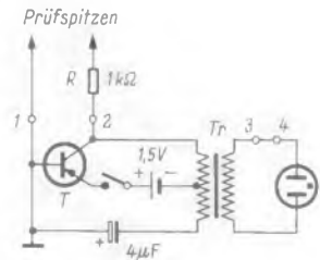
Schaltung eines Durchgangsprüfers mit Glimmlampe, bei dem die Glimmlampenspannung durch Transformation einer Tonfrequenzspannung gewonnen wird
