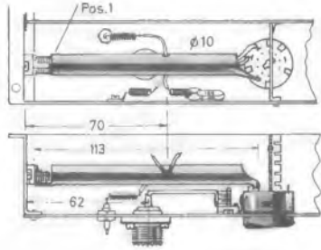
Bild 9. Konstruktion des Vorkreises
