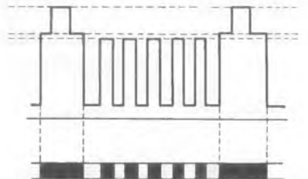
Bild 3c. Einwandfreie Impulsform des Signalgenerators. Das Signal muß bei fehlerfreiem Gerät in exakt rechteckiger Form an der Katode der Bildröhre meßbar sein
