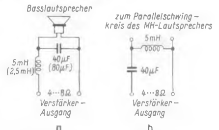
Bild 9. Schaltung der Frequenzweiche für den Tiefenbereich (a) und den MH-Bereich (b).
