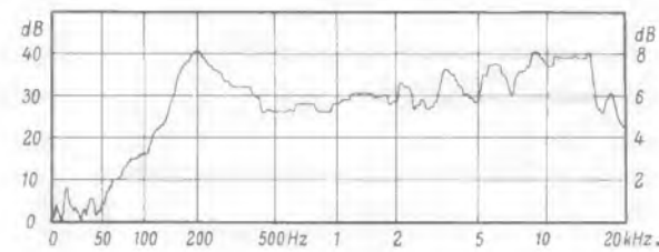
Bild 7. Schalldruck-Frequenzverlauf eines Einzelsystems P 10/Cl-13/65-10 000e Cu ohne Dämpfungstegen
