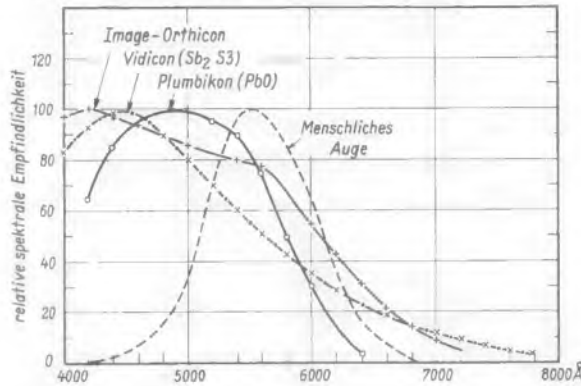
Unten: Bild 4. Relative spektrale Empfindlichkeit von drei bekannten Aufnahme- und des menschlichen Auges
