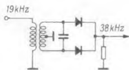
Bild 8. Verdoppeln der Pilotfrequenz mit Hilfe einer Doppelweg-Gleichrichtung
