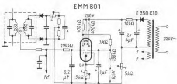
Bild 4. Ein unsymmetrischer Ratiodektor erfordert für diese Abstimmanzeige ein eigenes erdfreies Netzteil
