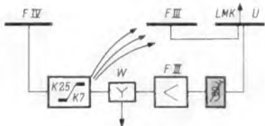
Der durch graue Tönung gekennzeichnete Sperrkreis für Kanal 7 unterdrückt die eingestrahelte Störung des Umsetzers
