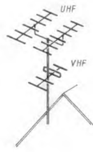
Links: Das Zusammenschalten zweier UHF- und einer VHF-Antenne für zwei Teilnehmer (A und B) mit Hilfe einer Verzweigungsdose V und zweier Weichen W. Rechts: Montage der drei Antennen an einem Mast
