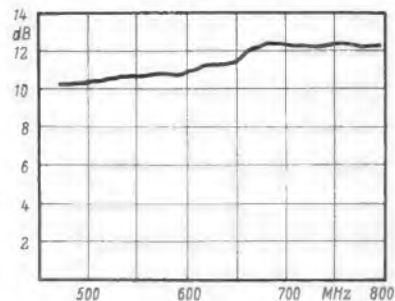
Bild 10. Verlauf des Gewinns des neuen Achterfeldes für 470...790 MHz (Fuba)
