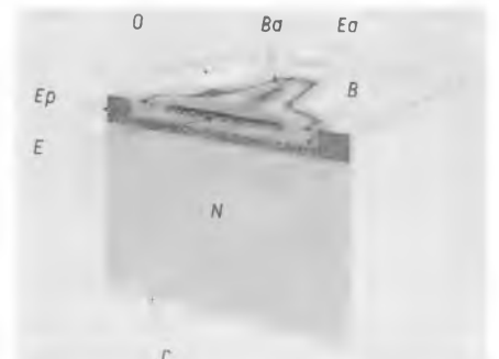
Bild 1. Sterngeometrie des Epitaxial-Planar-Transistors (von innen nach außen: Emitter, Basis, Kollektor)
