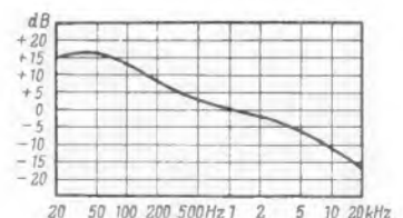
Bild 5. Frequenzkurve des Vorentzerrers PV 8
