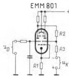
Rechts: Bild 2. Grundsätzliche Schaltung der Abstimmanzeigeröhre EMM 801
