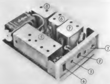
Bild 6. Innenansicht des Mikroport-Taschenempfängers Ela T 203 (Telefunken); 1 = Ein/Aus und Lautstärke; 2 = Buchse für Kleinhörer; 3 = Antennen-Gewindebuchse; 4 = Umschalter für Festfrequenzen 36,7 MHz und 37,1 MHz; 5 = Mischstufe; 6 = Zf-Stufe, 7 = Zf-Stufe und Regelleistungserzeugung
