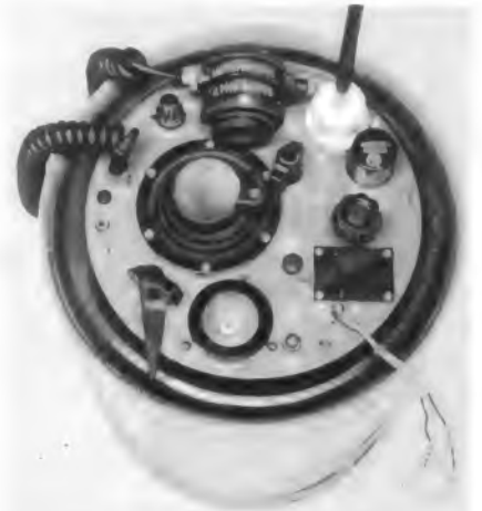
Bild 7. Blick auf die Bedienungsplatte der tragbaren Rettungsbootfunkstation SE 662 (Telefunken)
