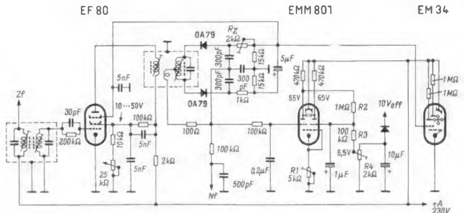
Bild 3. Begrenzerstufe und Ratiodektor eines UKW-Empfängers. Die Röhre EMM 801 zeigt den Nulldurchgang und die EM 34 die Summenspannung an
