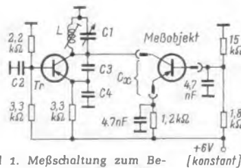
Bild 1. Meßschaltung zum Bestimmen kleiner Kapazitäten
