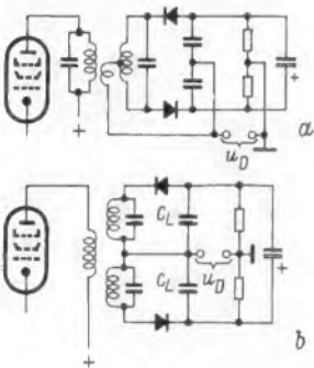
Links: Bild 1. a = Schaltung eines symmetrischen Ratiodektors, b = umgezeichnet als Ersatzschaltung von Bild a
