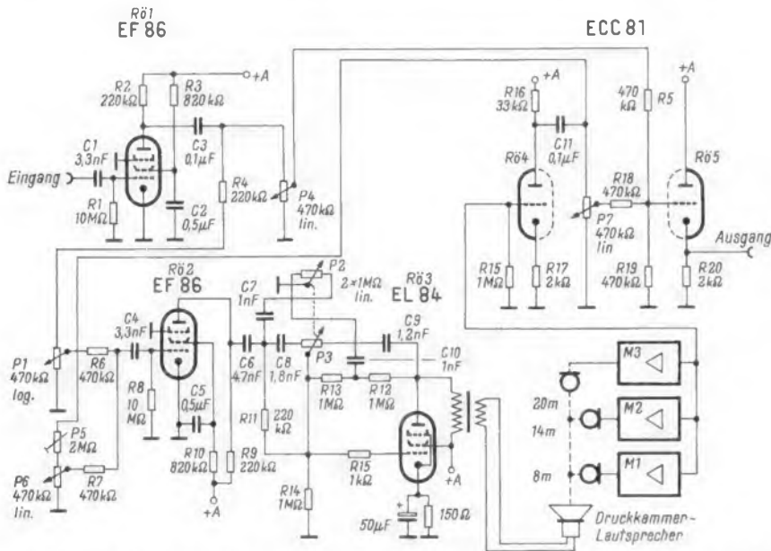
Bild 1. Gesamtschaltung des Nachhallgerätes. Die drei Mikrofonvorverstärker M 1 bis M 3 werden nach Bild 3 geschaltet
