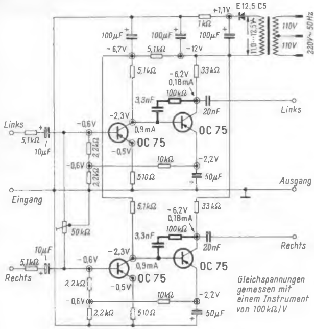
Bild 6. Schaltung des Transistor-Vorentzerrers
