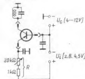
Bild 1. Meßschaltung zum Bestimmen kleiner Kapazitäten
