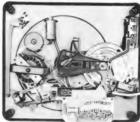
Bild 2. Unteransicht der Platine
