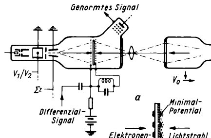
Bild 3. Gedächtnisröhre. a = Röhre zur Umwandlung des Differentialsignals in ein genormtes Signal, b = vergrößertes Ausschnitt der Speicherfläche. Rechts die Lichtstrahl-Abströhre
