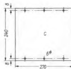
Bild 4. Schablone aus Preßpappe für das exakte Bohren der Wände
