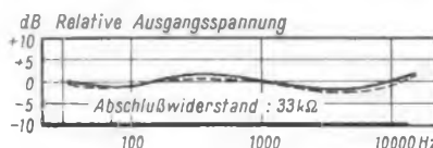
Bild 3. Frequenzkurve des Stereo-Abtastsystems STS 220 D bezogen auf konstante Auslenkgeschwindigkeit; relative Ausgangsspannung in dB, Abschlußwiderstand = 33 kΩ, Auflagekraft = 4 p, Meßschallplatte Westrex 1 A
