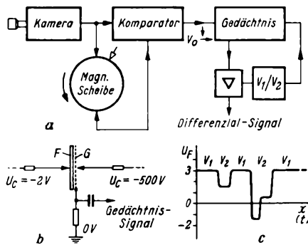
Bild 2. Differential-Bildwähler (Sender). a = Weg zwischen Kamera und Sender, b = Gedächtnis-Vorrichtung, c = Geschwindigkeitswechsel der Abtastung des Gedächtnisses
