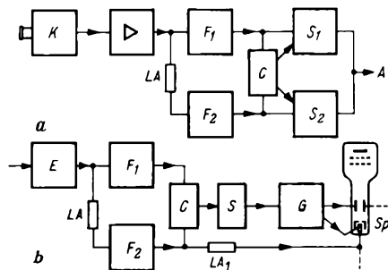
Bild 4. Prinzip der Frequenzbandkompression mit automatischer Messung des „Detailfaktors“. a = Sender (K = Kamera, LA = Verzögerungsleitung, F 1 , F 2 = Tiefpässe, C = Komparator, S 1 , S 2 = Umschalter); b = Empfänger (E = Eingangsschaltung, G = Fernsehempfänger, S = Schalter, Sp = Speicherrohre, sonst wie unter a)
