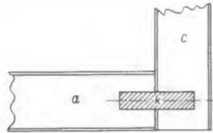
Bild 3. Eine Verbindungsstelle der Preßspanplatten im Schnitt, die Buchstaben entsprechen denen von Bild 2
