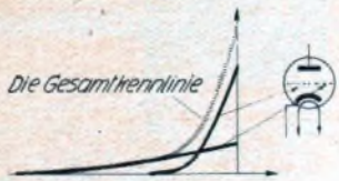
Abb. 3. Die Gesamtkennlinie einer Regel-Dreipolröhre setzt sich aus zwei Einzelkennlinien zusammen.
