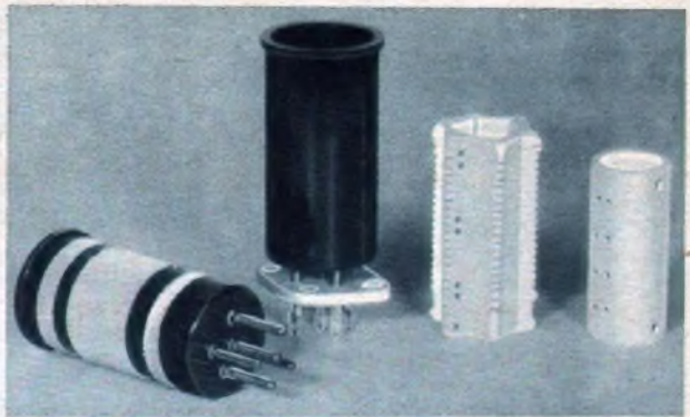
Abb. 7. Einige Kurzwellen-Spulen-körper. Archivbild.
