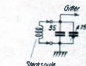
Abb. 5. Die einfachste und beste Schaltung zur Bandabstimmung; Festkondensator mit parallelem Abstimm-Drehko.
