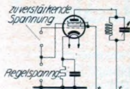
Abb. 4. Die 6-Polregelröhre und ihre Schaltung.
