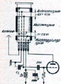
Abb. 6. So sind zweckmäßig bei einer flexiblen Kurzwellen-Spule die Windungen aufzubringen und die Anschlüsse zu legen.
