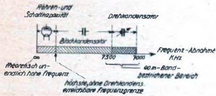
Abb. 4. Das Prinzip der Bandabstimmung mit Berücksichtigung der Schaltkapazitäten.
