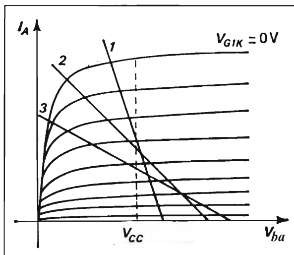
figura 3: distorsione in un pentodo a seconda del carico dinamico
