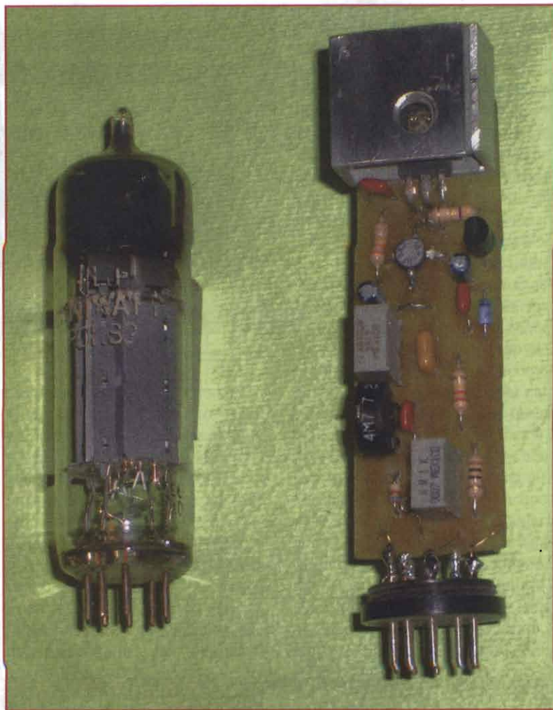
figura 1: la valvola Noval (a sinistra) ed il suo "clone"
