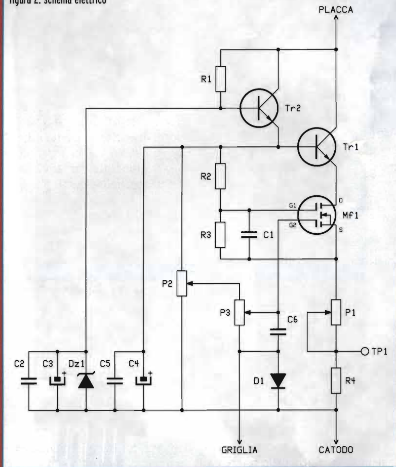
figura 2: schema elettrico
