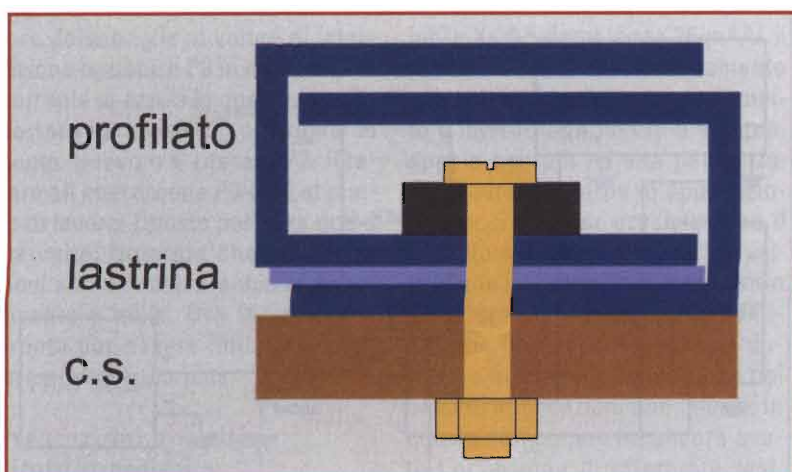
figura 4: disposizione del dissipatore
