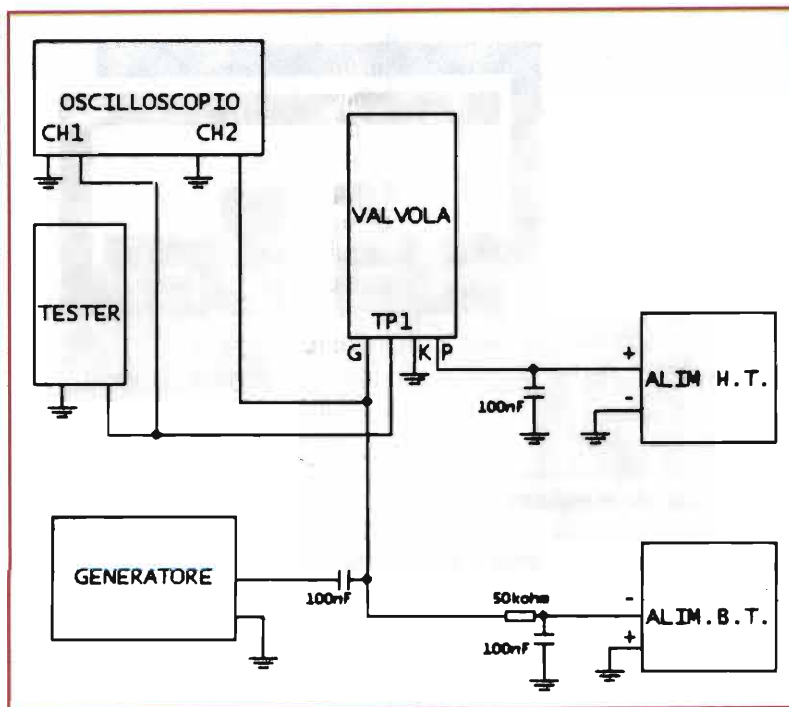
figura 5: disposizione strumenti per la taratura al banco
