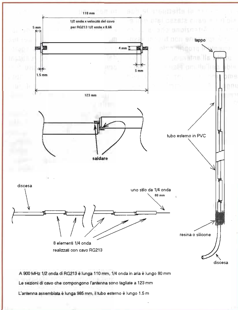
figura 1: sequenza di montaggio della collineare a 900 MHz
