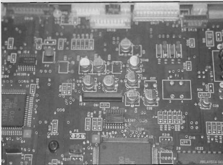
Foto 3 - I condensatori SMD responsabili del...primo problema
