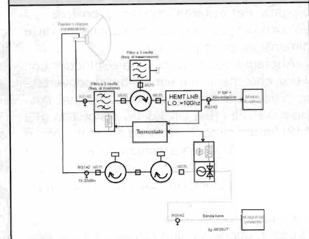
Sistema definitivo di conversione 10GHz (con TX a diodo Gunn).
