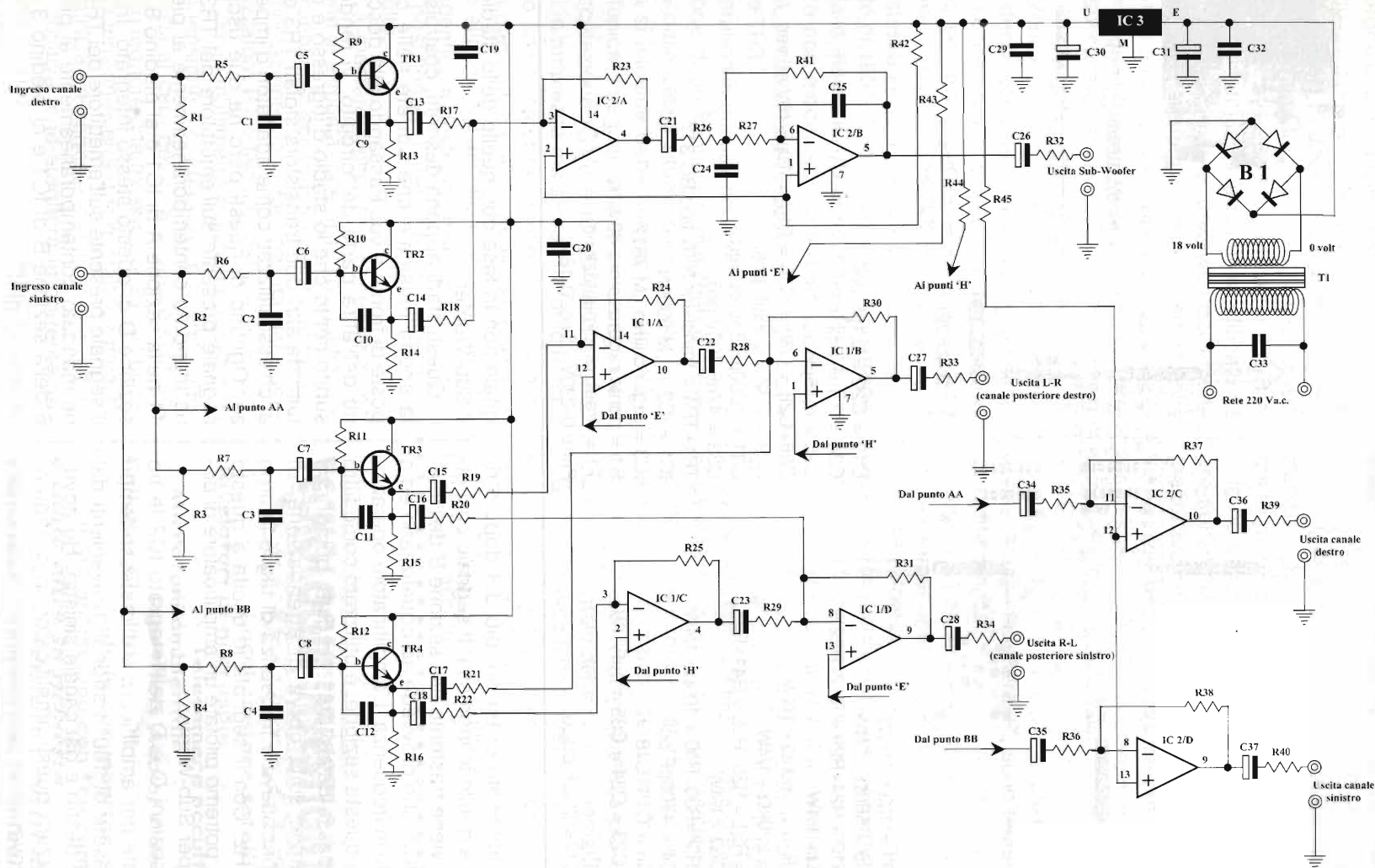
Schema elettrico
