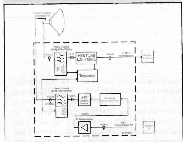
Sistema iniziale di conversione 10GHz (con TX a moltiplicatore).
