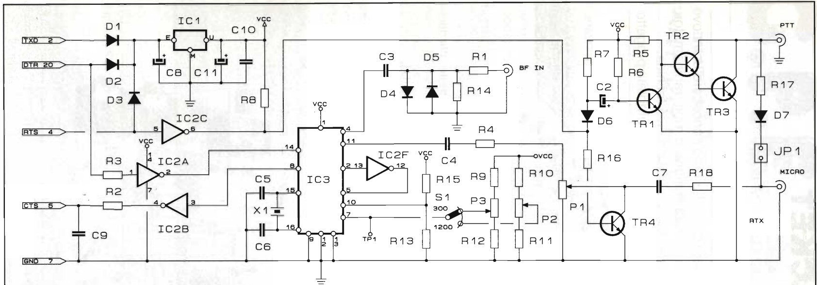
figura 1 - Schema elettrico.
