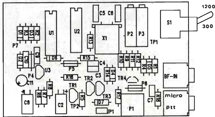
figura 2 - Disposizione componenti.
