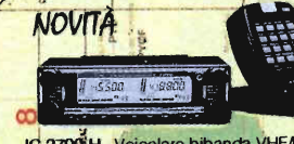
IC 2700 H - Veicolare bibanda VHF/UHF Tx: 144/146 - 430/440 MHz Rx: 118/174 - 320/470 MHz Conferma ricezione da 830 a 950 MHz
