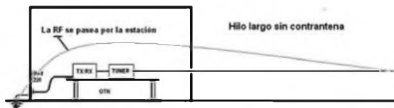
Figura 2 - Hilo Largo sin contra-antena
