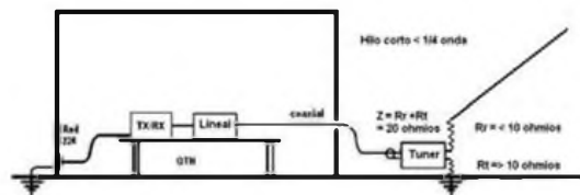
Figura 3 - Hilo Corto con toma de tierra
