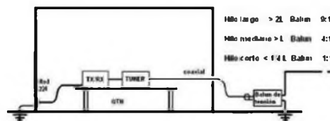
Figura 7 - Hilo Largo Con Balun 9:1 o 4:1 0 1:1
