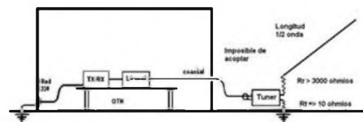
Figura 4 - Hilo Corto de media onda
