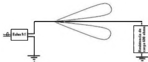
Figura 10 - Diagrama de radiación de antena Beverage
