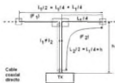
Figura 4 - Dipolo con cable coaxial directo
