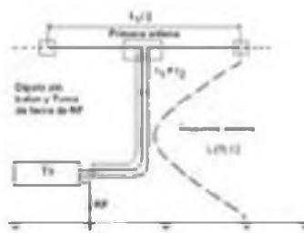
Figura 10 - Dipolo sin balun y con toma de tierra de RF
