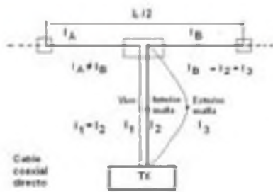
Figura 3 - Dipolo con cable coaxial directo = 3 conductores
