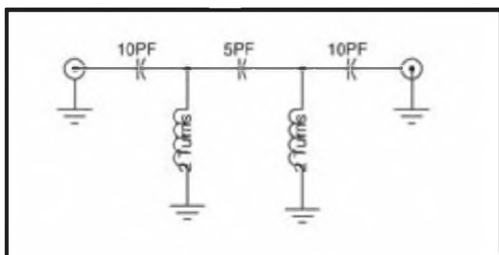
Figura 2. Esquema de un filtro paso alto de 2 etapas
