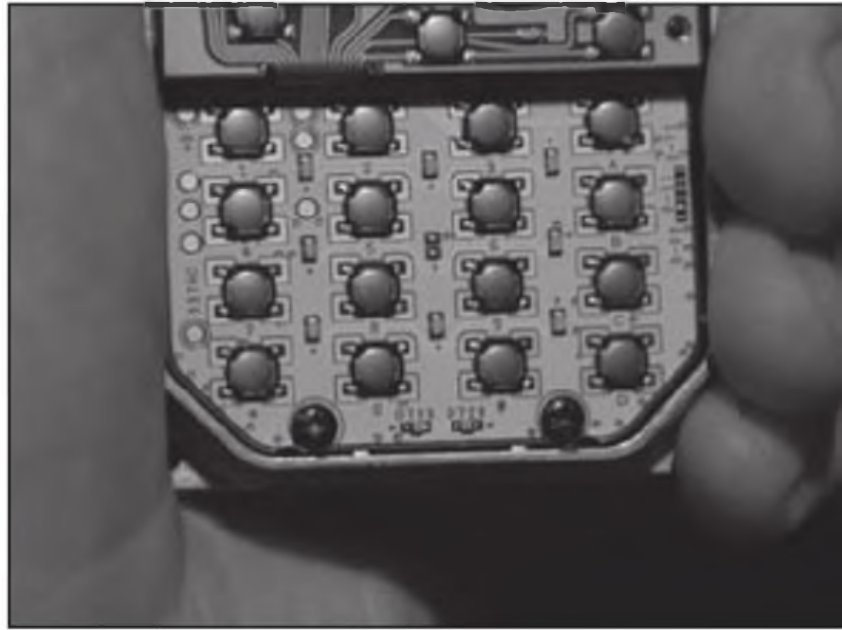
Foto F. El teclado del D-72 se puede reemplazar fácilmente si se estropea. Es muy fácil extraer el viejo y encajar uno nuevo.
