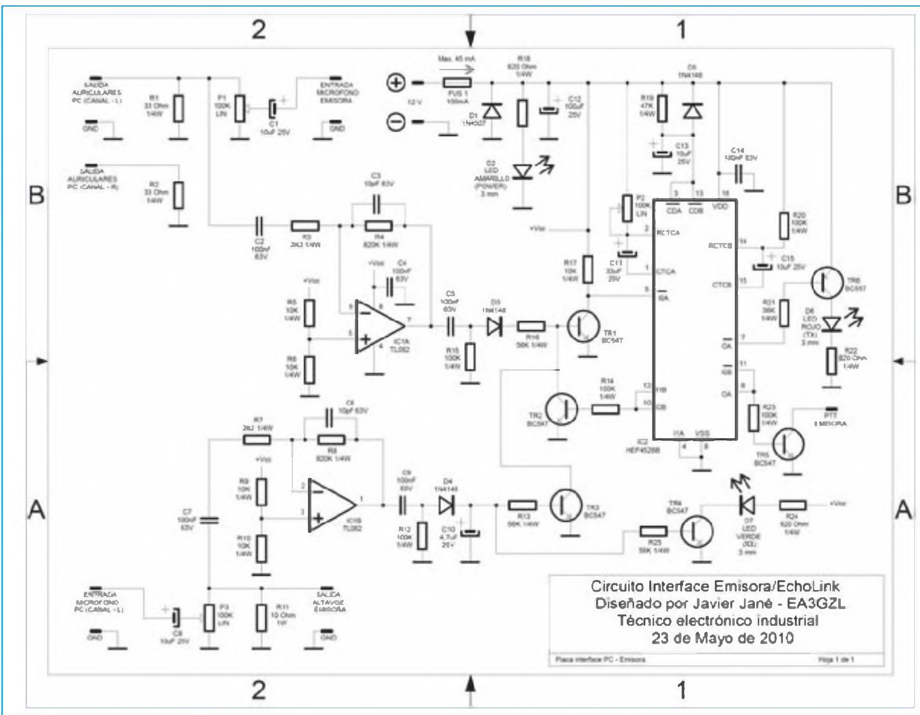
Figura 1. Esquema general de la interfaz EchoLink.
