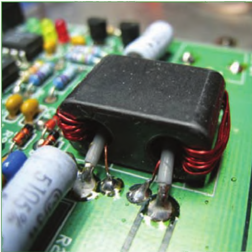
Foto A. Toroide tipo "binocular". Es más fácil de bobinar de lo que parece.
