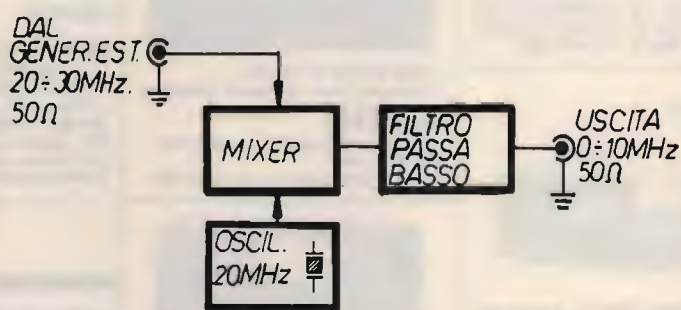
figura 1 Schema a blocchi del Converter.
