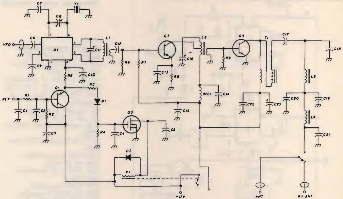
figura 2 Schema elettrico del transceiver sezione trasmettitore.
