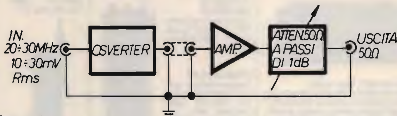
figura 2 Osverter ampliato.
