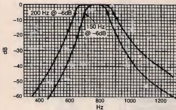
figura 2 Curva di risposta del filtro CW.
